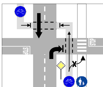
1. ábra. A felsőbbrendű úttal párhuzamosan haladóknak elsőbbség van a kanyarodó ill. keresztbe közlekedő járművekkel szemben.
